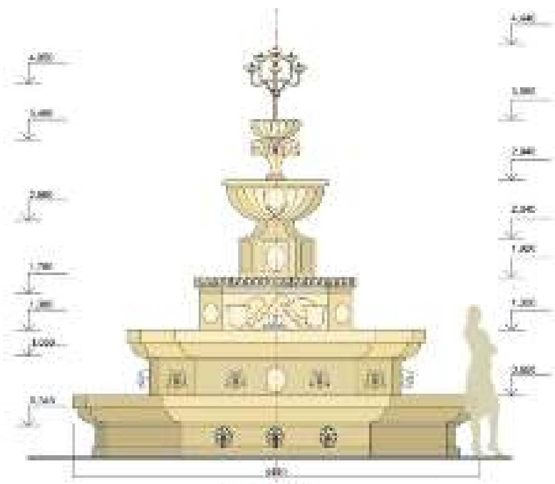
Рисунок 1-1 М 1:20
